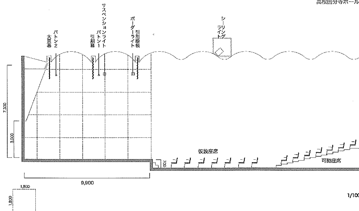
舞台断面図
