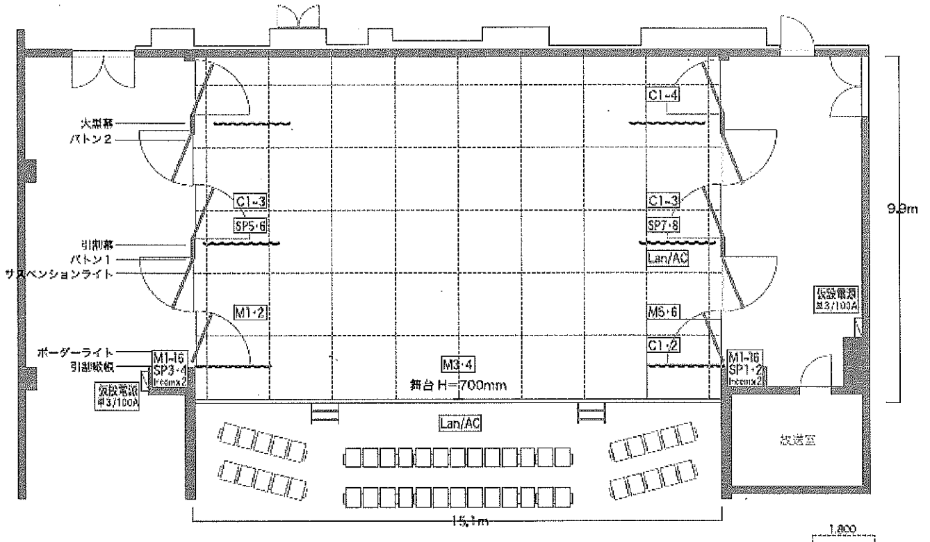
平面図
